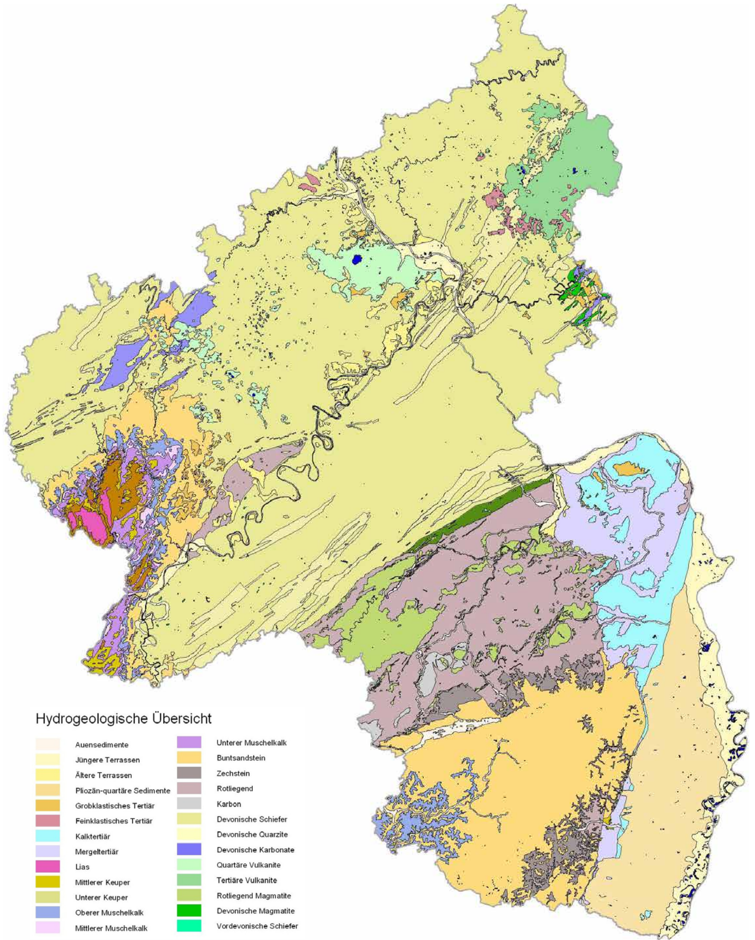
Abb. 1: Hydrogeologische Einheiten in Rheinland-Pfalz (HÜK 300, Landesamt für Geologie und Bergbau Rheinland-Pfalz)
