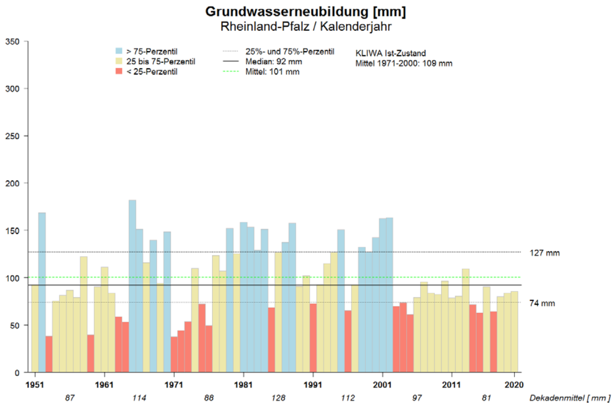
Abb. 8: Mittlere jährlichen Grundwasserneubildungshöhe der Reihe 1951 - 2020
